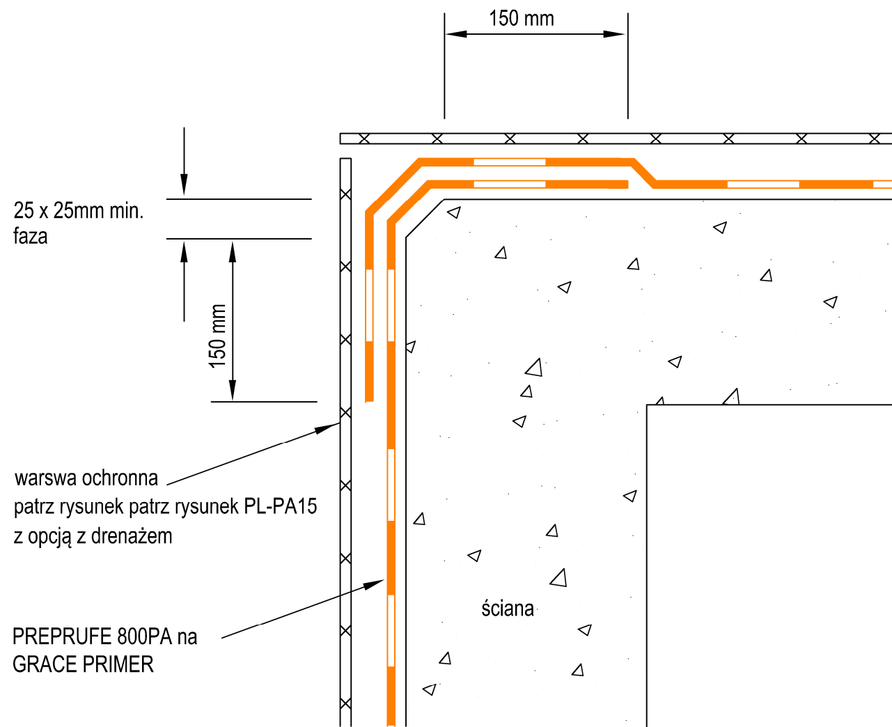
NAROŻNIK ZEWNĘTRZNY PIONOWY RZUT
