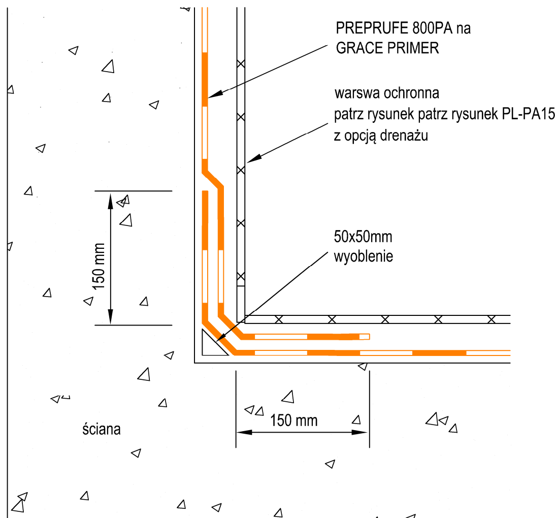
NAROŻNIK WEWNĘTRZNY PIONOWY RZUT
